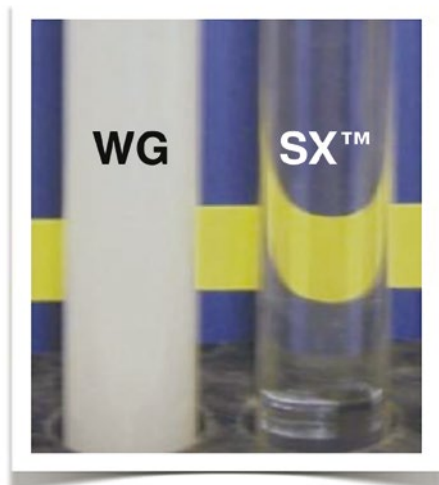
Rozpuszczalność formacji SX w stosunku do formacji WG
